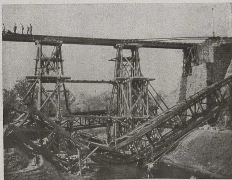
Die von den Russen gesprengte und von uns wiederhergestellte Eisenbahnbrücke bei Radymno (10. Juni 1915)
